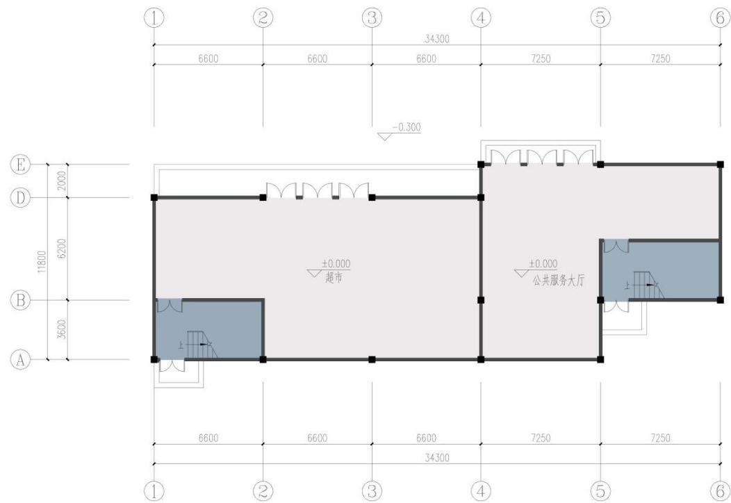
一层平面图
