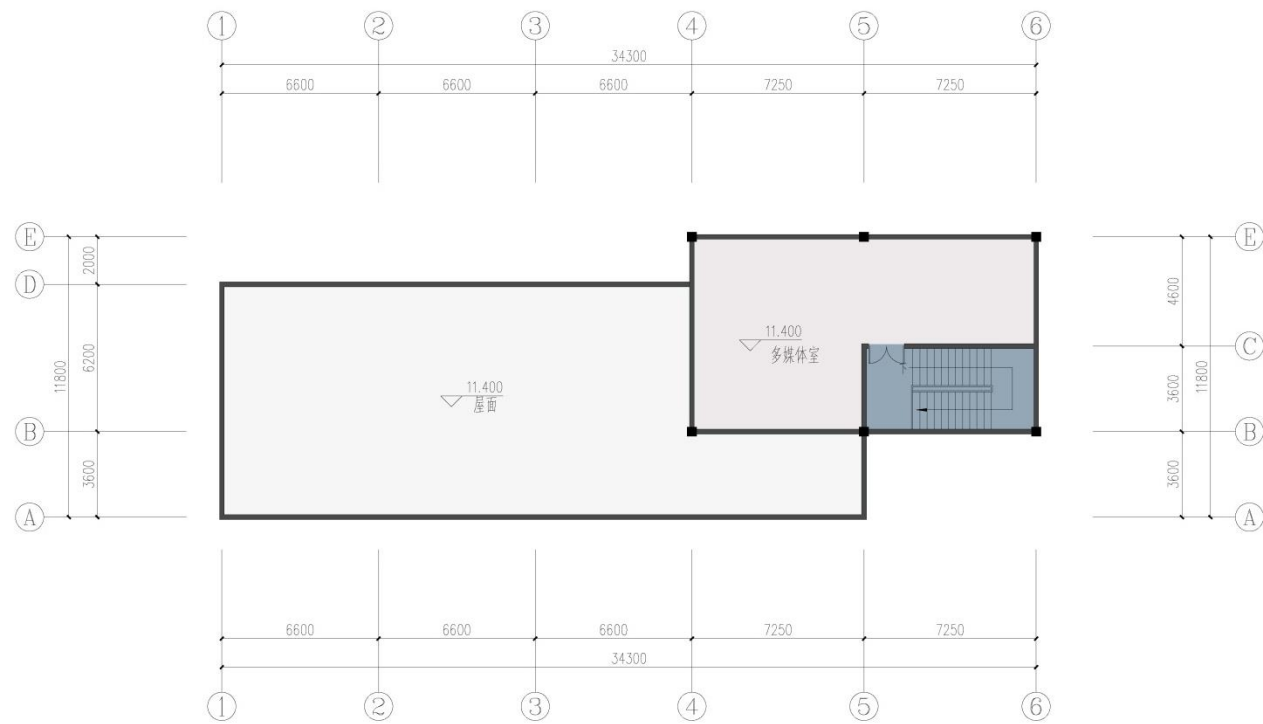
三层平面图
